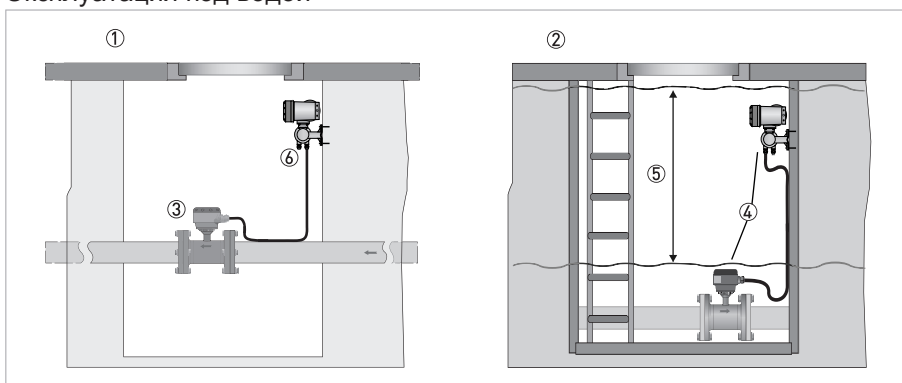
Рисунок 3-16: Примеры монтажа в измерительном колодце
