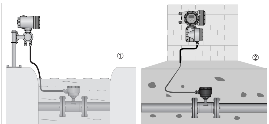
Рисунок 3-15: Примеры применений на подтопляемых территориях и под землей
