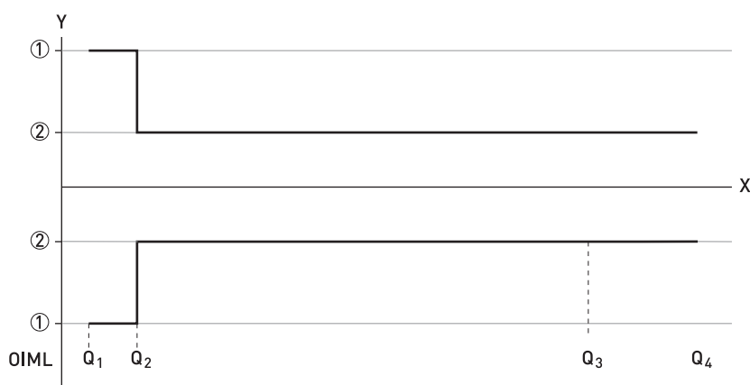
Рисунок 2-1: Расходы согласно стандарту ISO добавлены к рисунку для сравнения со стандартом OIML.
