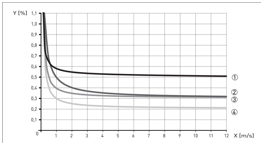
Рисунок 2-3: Зависимость погрешности измерений от скорости потока X [м/с]: скорость потока Y [%]: отклонение от актуально измеренного значения (ИЗ)
