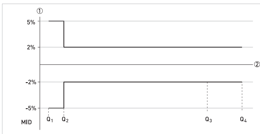
Рисунок 2-2: Расходы согласно стандарта Международной организации по стандартизации (ISO) добавлены к рисунку для сравнения с Директивой по измерительному оборудованию (MID)
