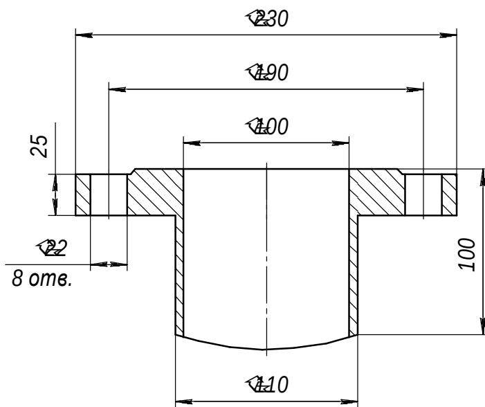
Размеры приварного патрубка на давление 2,5 и 4,0 МПа
